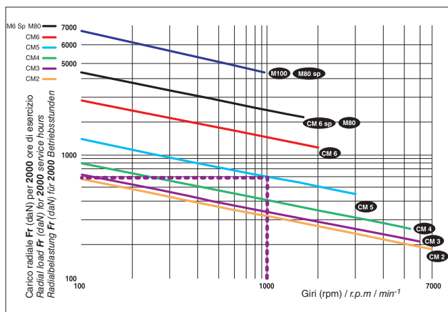
MOD. M Carico radiale / Radial load / Radialbelastung
